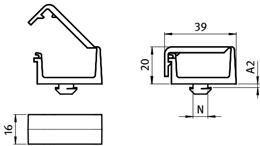
Clip-Kabelbinder mit Hammer Clip Cable Binder with Hammer
